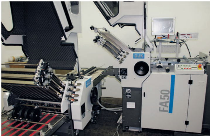
Für minimale Falzgrößen bis 15 mm, für Altarfaltungen oder Flyer etc. ist die GUK FA50/6 und das zweite Werk FA35/6 bei Druck-Kultur bestens geeignet.
